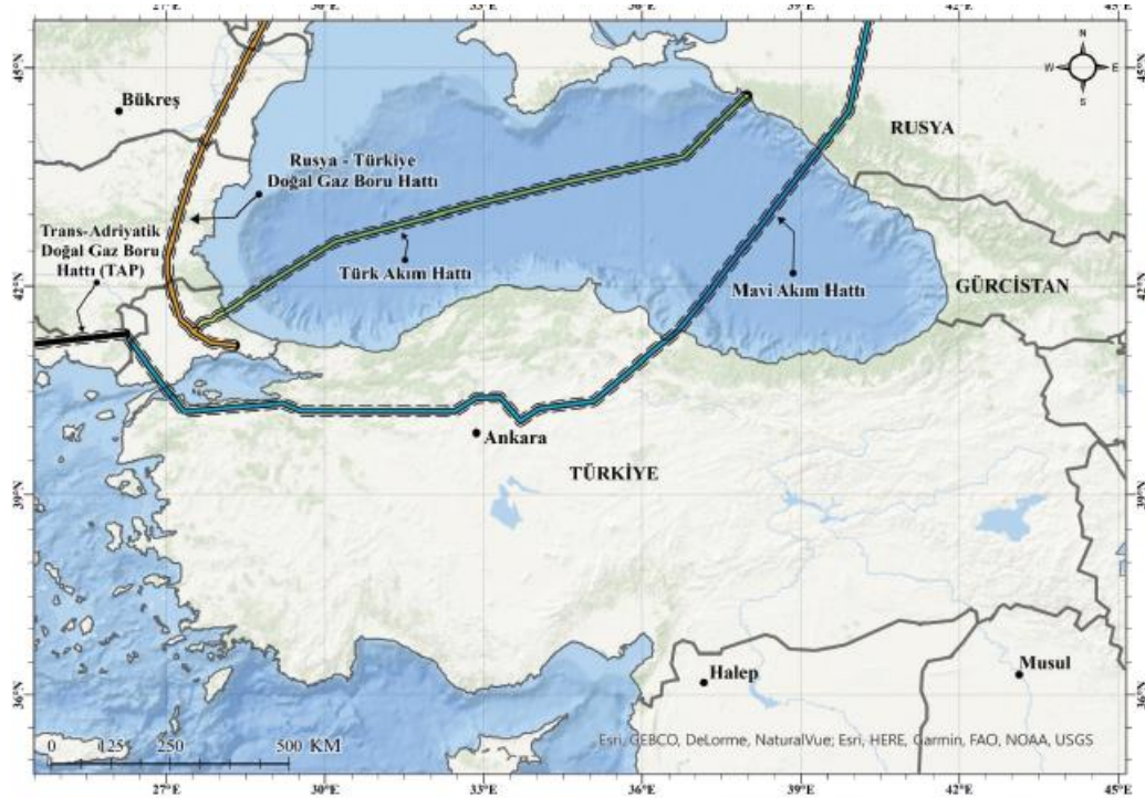
Şekil-2: Karadeniz Havzası'ndaki Doğal Gaz Boru Hatları 19
